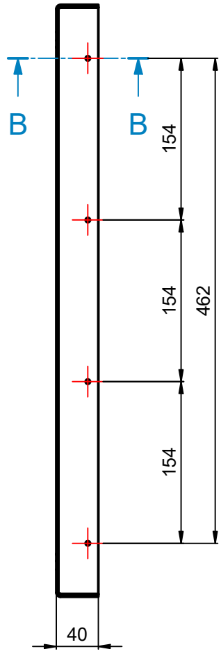
A-A (1 : 5)
