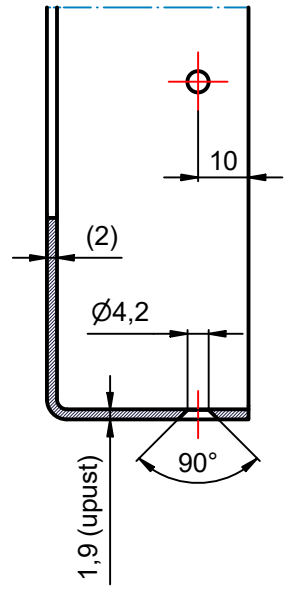
B-B (1 : 1,5)
